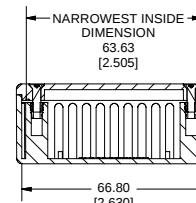
SECTION D-D
